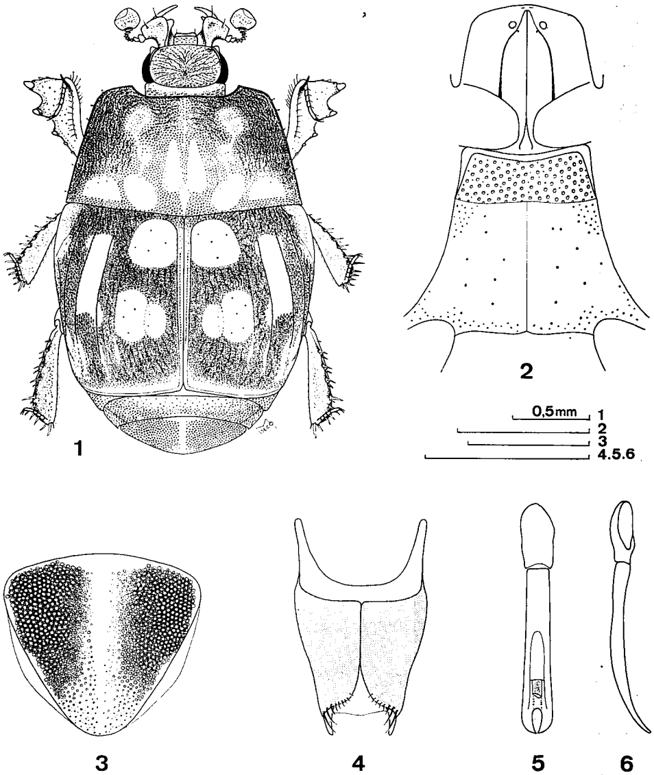
Fig. 1 à 6: Dahlgrenius mirificus n. sp. — Fig. 1: habitus ♂. — Fig. 2: pro-mésomé-tasternum. — Fig. 3: pygidium. — Fig. 4: huitième urosternite ♂ en vue ventrale. — Fig. 5: édéage en vue dorsale. — Fig. 6: édéage en vue de profil.
