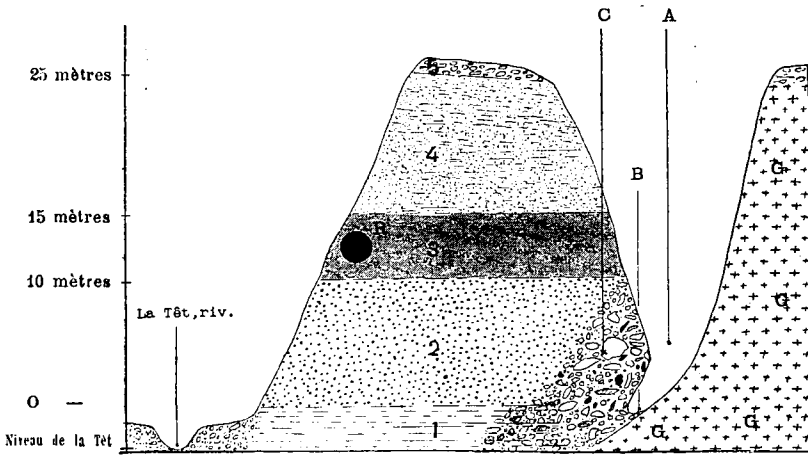
FIG. 1. — Coupe du Plaisancien à Millas (lieu dit « Coume d'al Douc »).
