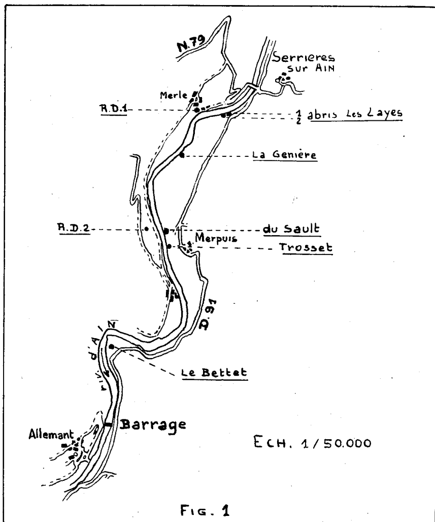
Situation des gisements de la basse vallée de l'Ain entre Serrières-sur-Ain et Allemant.
