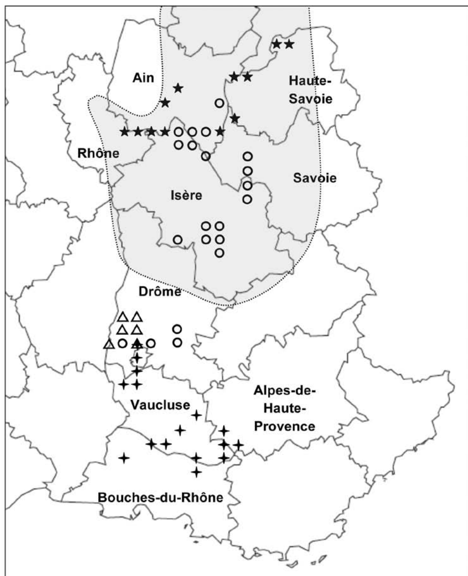
Figure 1 – Répartition des Ophrys cf. fuciflora , dans le quart sud-est de la France, d'après Dusak & Prat (2010), Martin & Véla (2012) et les observations des auteurs. Quadrillage Lambert 93, un point pour 10 x 10 km.
