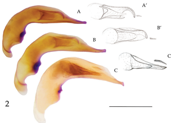
Figure 2 – Pièces génitales mâles (lobe médian en vue latérale) : (A) Trechus lallemantii de Dardara (Rif, Maroc) ; (B) Trechus zorgatii n. sp. du système karstique du Kef Chgeg (Tunisie) ; (C) T. djbelgloubensis n. sp. du Djbel Gloub (Tunisie).
