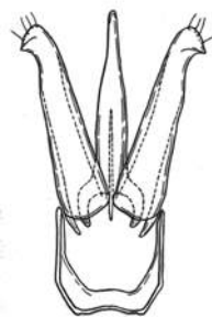
Fig. 1 : Athous kruegeri Reitter, habitus – Fig. 2 : Athous jarrigei nov. sp., habitus – Fig. 3 : Athous jarrigei nov. sp. : front vu de dessus – Fig. 4 : Athous jarrigei nov. sp., front : creux médian – Fig. 5 : Athous kruegeri Reitter : édage – Fig. 6 : Athous jarrigei nov. sp. : édage (dessin Leseigneur 1972, fig. 237 p. 207).
